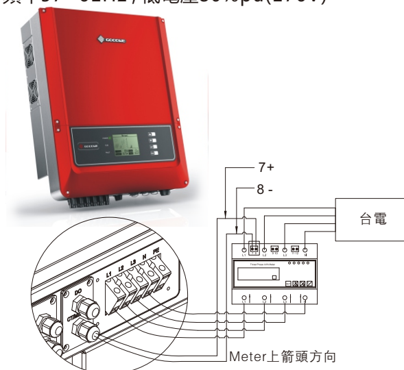
防逆流偵測器訊號線接孔
